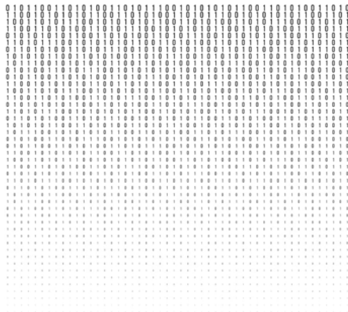
Binär-code
