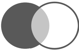
Figur I (Venn-Diagramm). 65
