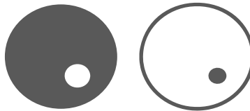
Figur III (Strikte Antinomie)
